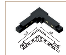
48V-Q1 CONNECTOR MINI
