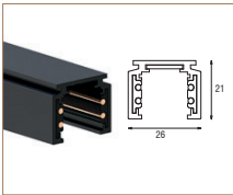
48V-Q1 SURFACE MINI TRACK RAIL
